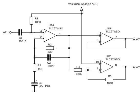
Rysunek 6. Schemat ideowy stopnia wejściowego ze wzmacniaczami operacyjnymi
