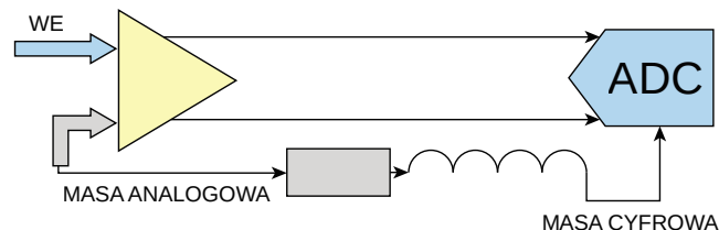
Rysunek 1. Wyjaśnienie drogi propagacji zakłóceń przez masę w układzie ze wzmacniaczem typu single-ended
