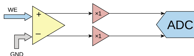
Rysunek 2. Schemat blokowy stopnia wejściowego ze wzmacniaczem różnicowym
