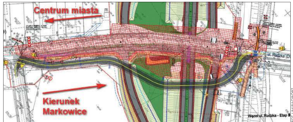
Schemat nowej organizacji ruchu w rejonie kanatu Ulgi w Raciborzu. Wyjazd w kierunku Markowic oraz dojazd do centrum odbywa się po drodze tymczasowej.
