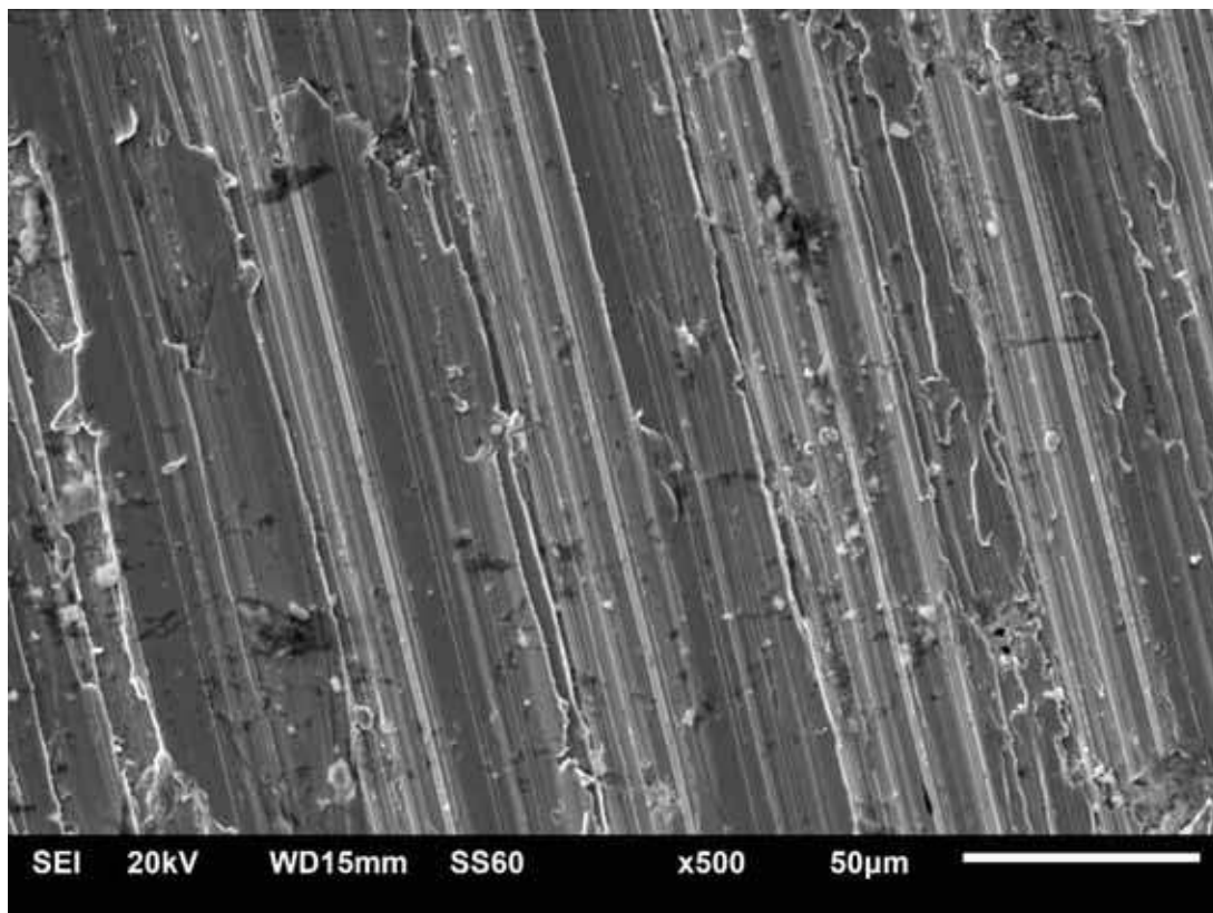
Ostrogę z Narzymbia badano metodą SEM na podstawie sygnału pochodzącego z elektronów wtórnych. Na zdjęciu badany obszar ostrogi
