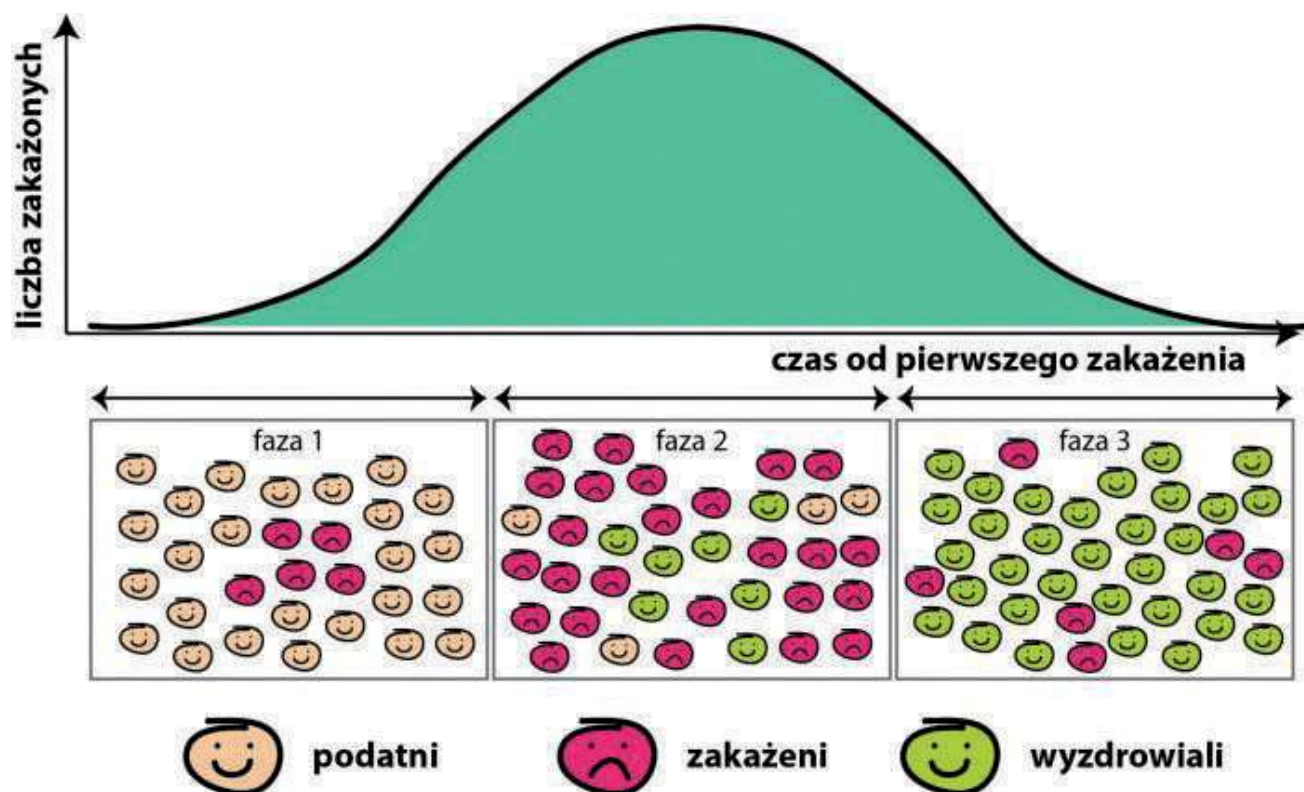
Wykres 1. Krzywą epidemiologiczną można podzielić na trzy fazy. W fazie 1. następuje wykładniczy przyrost zakażonych, ponieważ populacja jest podatna na chorobę (nie ma odporności). W fazie 2. epidemia spowalnia, bo liczba osób podatnych maleje i większość z nich jest albo zakażona, albo odporna. W fazie 3. fala mija, gdy nowych zakażonych nie przybywa a populacja zdrowieje.
