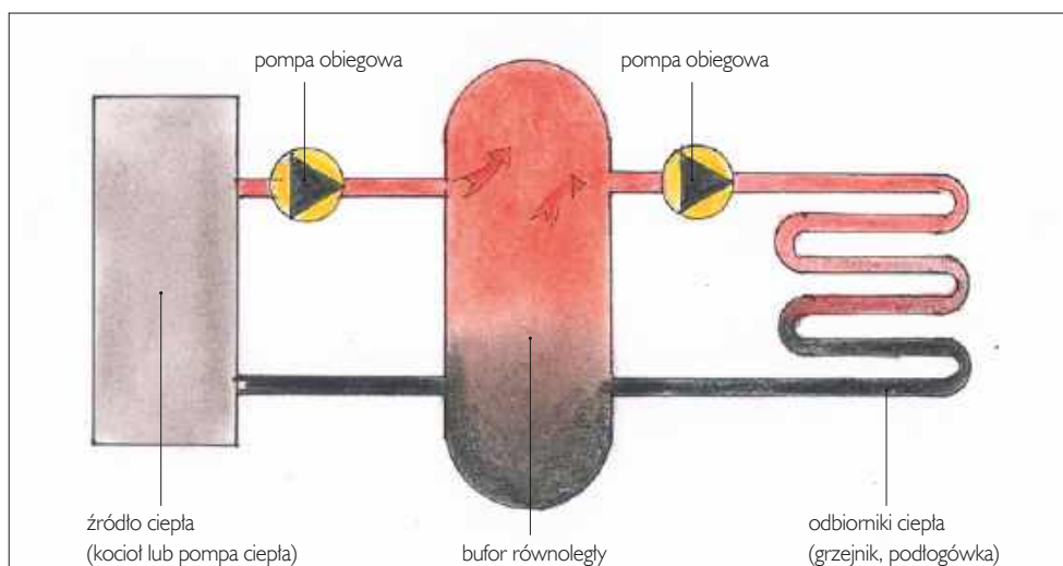
➊ Bufor równoległy uniezależnia przepływ wody przez kocioł (źródło ciepła) oraz przez resztę instalacji grzewczej.
