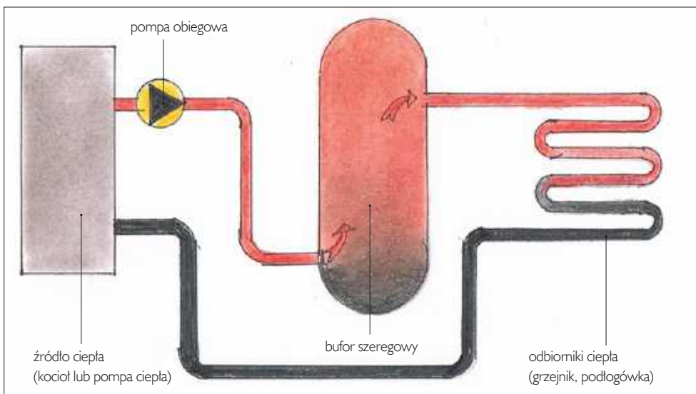
➋ Bufor szeregowy zwiększa jedynie zbiór wody. Jej przepływ przez instalację oraz kocioł lub pompę ciepła zawsze musi następować równocześnie.
