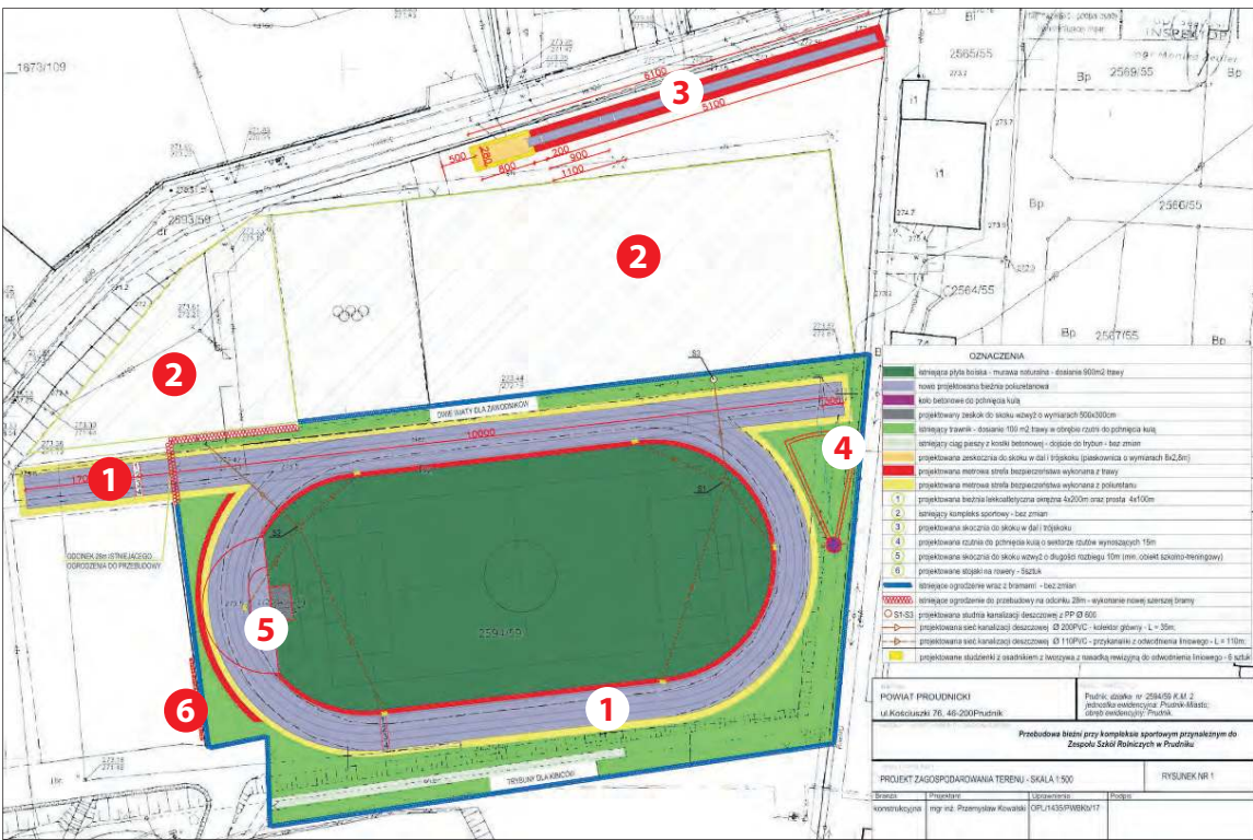
Plan wizualny inwestycji: 1 - projektowana bieżnia lekkoatletyczna okrężna (4x200m) i prosta (4x100m); 2 - istniejący kompleks sportowy; 3 - projektowana skocznia do skoku w dal i trójskoku; 4 - projektowana rzutnia do pchnięcia kulą; 5 - projektowana skocznia do skoku wzwyż; 6 - projektowane stojaki na rowery
