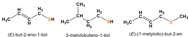
Rys. 1. Związki siarkowe o przykrym zapachu znajdujące się w wydzielinie skunksowatych.
