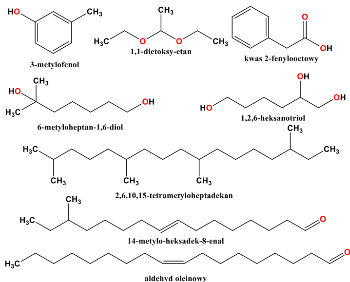
Rys. 2. Składniki piżma o charakterze węglowodorów, alkoholi, eterów, aldehydów i kwasów karboksylowych
