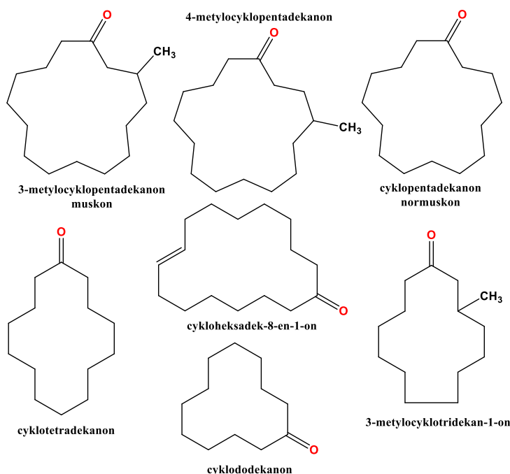
Rys. 3. Składniki piżma o charakterze makrocyclicznych ketonów.
