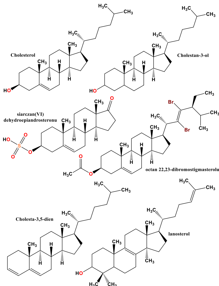
Rys. 4. Składniki piżma o charakterze steroidów i ich estrów.
