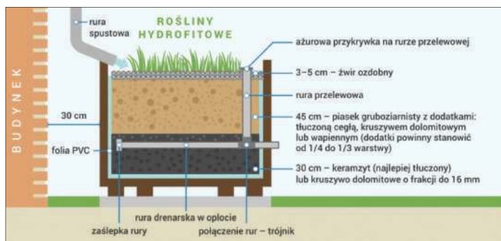
Ogród deszczowy w formie runda filtrującego – źródło: Fundacja Sendzimira ( https://sendzimir.org.pl )
