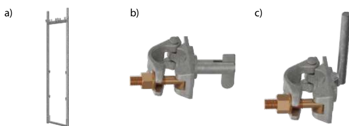
Rys. 4. Części składowe rusztowań ramowych umożliwiające montaż elementów dodatkowej balustrady: a) ramy z dodatkowymi elementami do montażu poręczy i krawężnika b) złącze poręczowe, c) złącze krawężnikowe
