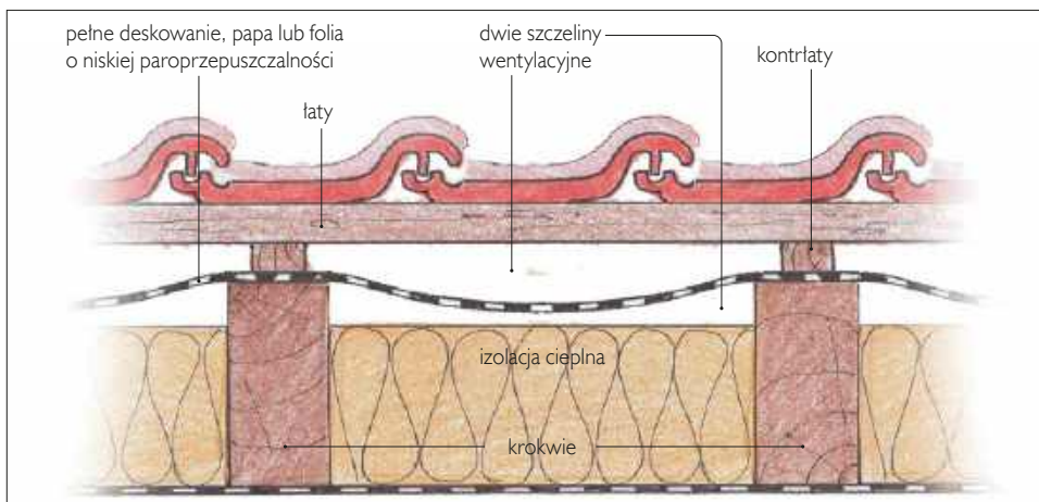
➋ Dwie szczeliny wentylacyjne – jedna pod pokryciem, druga nad ociepleniem – są niezbędne jeżeli wykorzystuje się folię dachową o niskiej paroprzepuszczalności, papę na deskowaniu, szczelne pełne deskowanie. Każdy z tych materiałów blokuje bowiem dalszy ruch pary wodnej.
