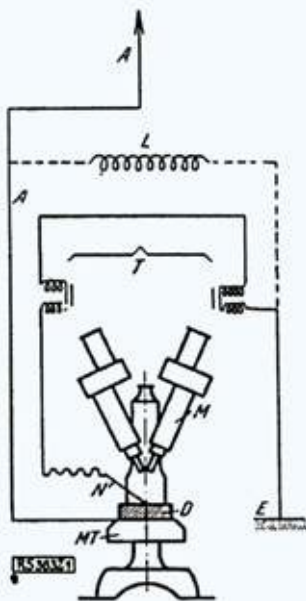
Schemat radiomikroskopu Czochralskiego
